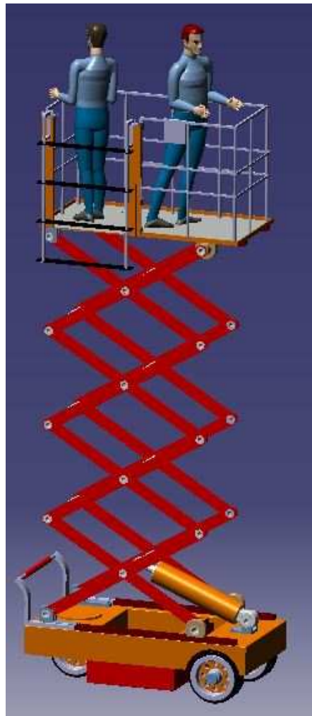
Figure4.1 Conception 3D sur CATIA V5
